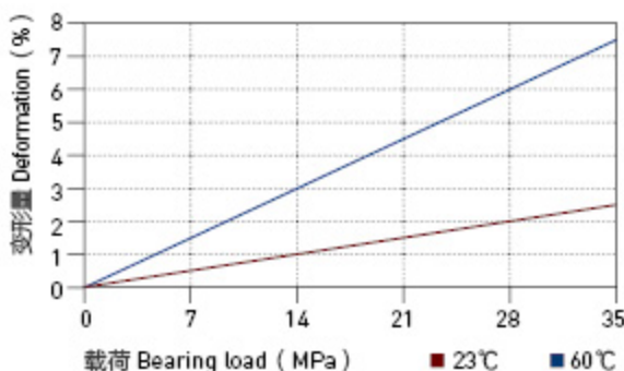
图表 HPP28-3: 载荷 - 温度图表
