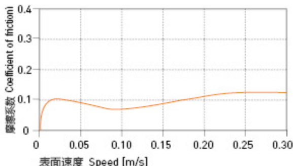
图表 HPP28-5: 摩擦系数与载荷变化关系图表 v=0.2m/s
