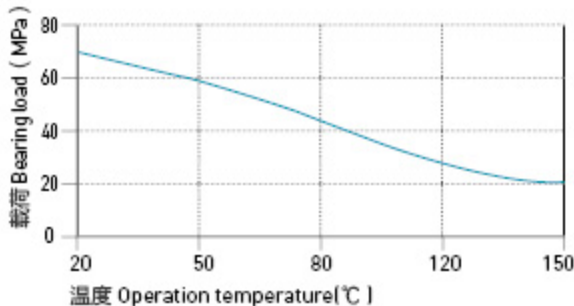
图表 HPP28-3: 载荷 - 温度图表
