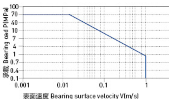
图表 HPP28-1: PV 图表
