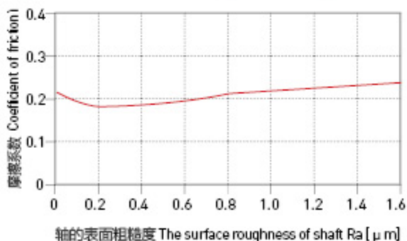
图表 HPP28-6: 摩擦系数与轴的表面粗糙度关系图表
