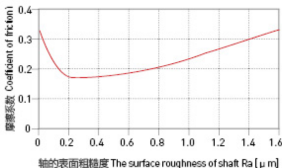
图表 HPP25-6: 摩擦系数与轴表面粗糙度关系图表
