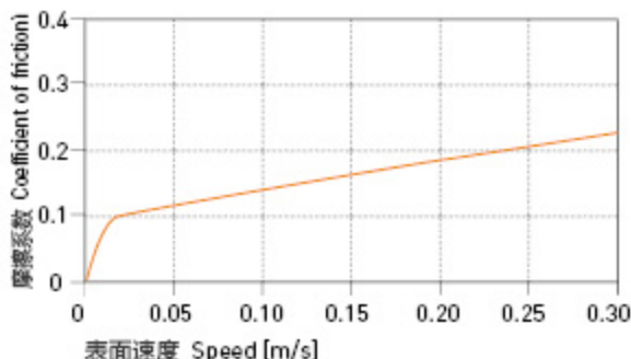
图表 HPP25-5: 摩擦系数与载荷变化关系图表 v=0.2m/s
