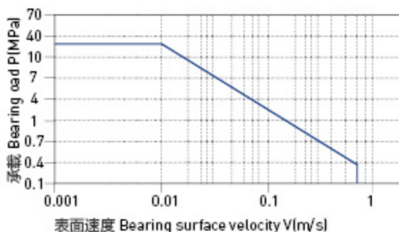
图表 HPP25-1: PV 图表
