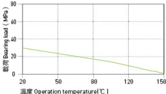
图表 HPP25-3: 载荷 - 温度图表
