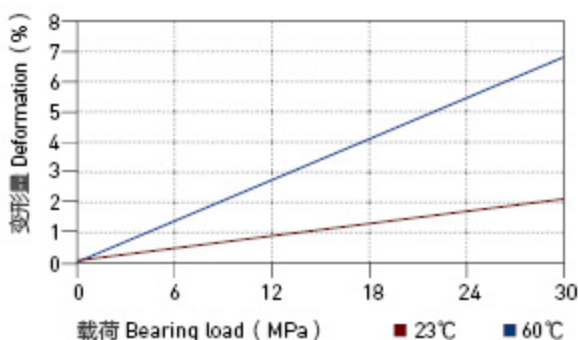
图表 HPP25-3: 载荷 - 温度图表
