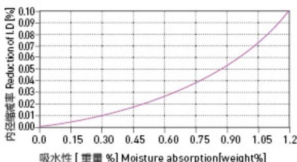
图表 HPP25-9: 吸水性的影响
